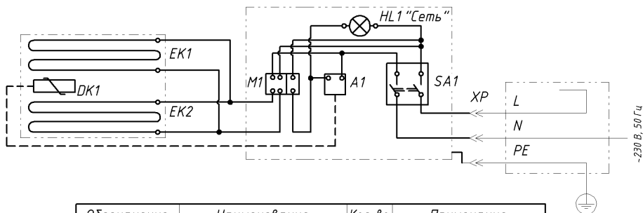
СХЕМА ЭЛЕКТРИЧЕСКАЯ ПРИНЦИПАЛЬНАЯ
